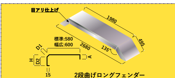
2段曲げロングフェンダー
