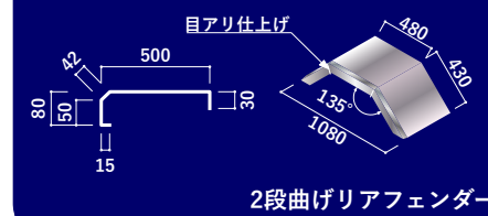
2段曲げリアフェンダー
